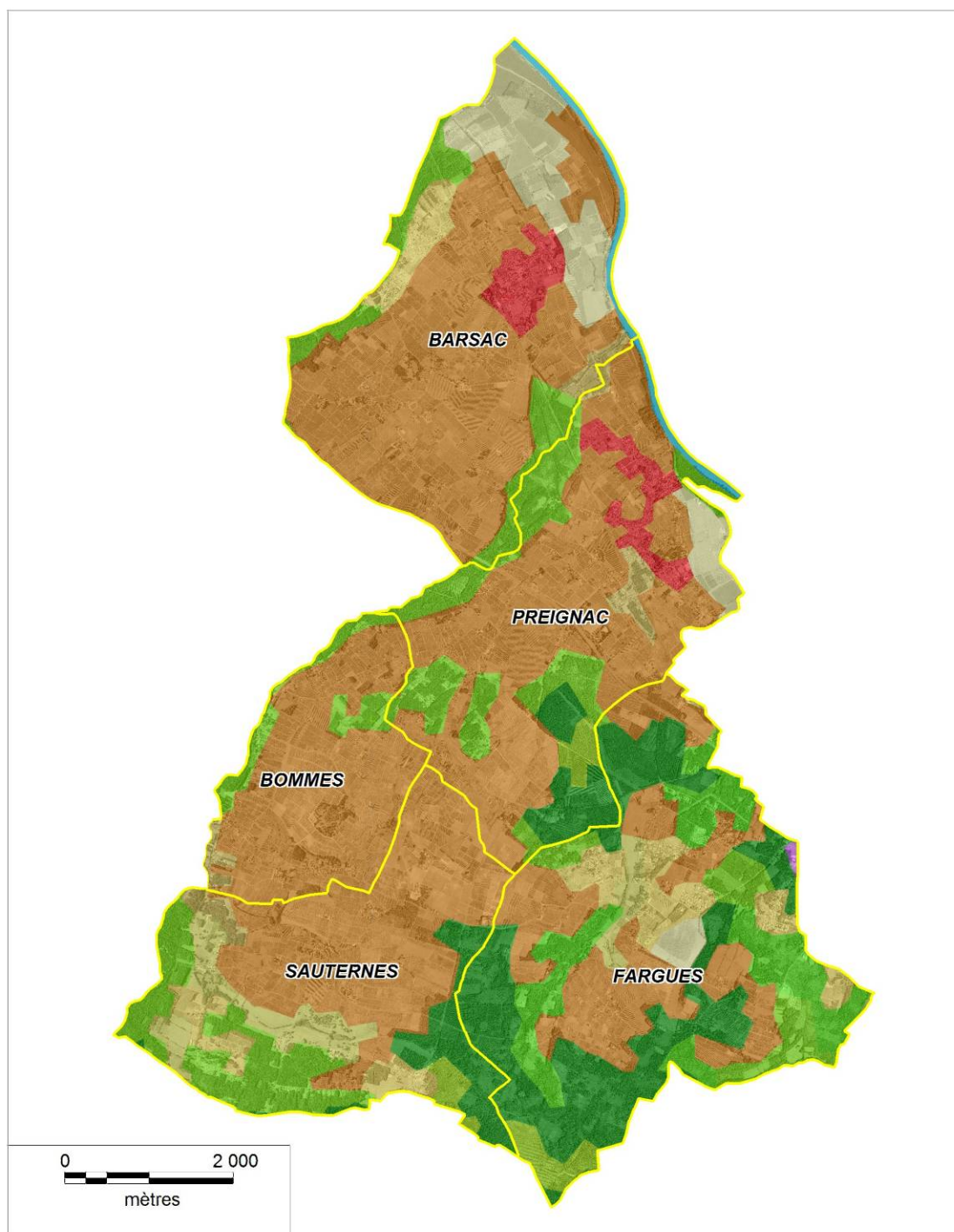
Carte 3 : Occupation du sol d'après la couverture Corine Land Cover 2006
