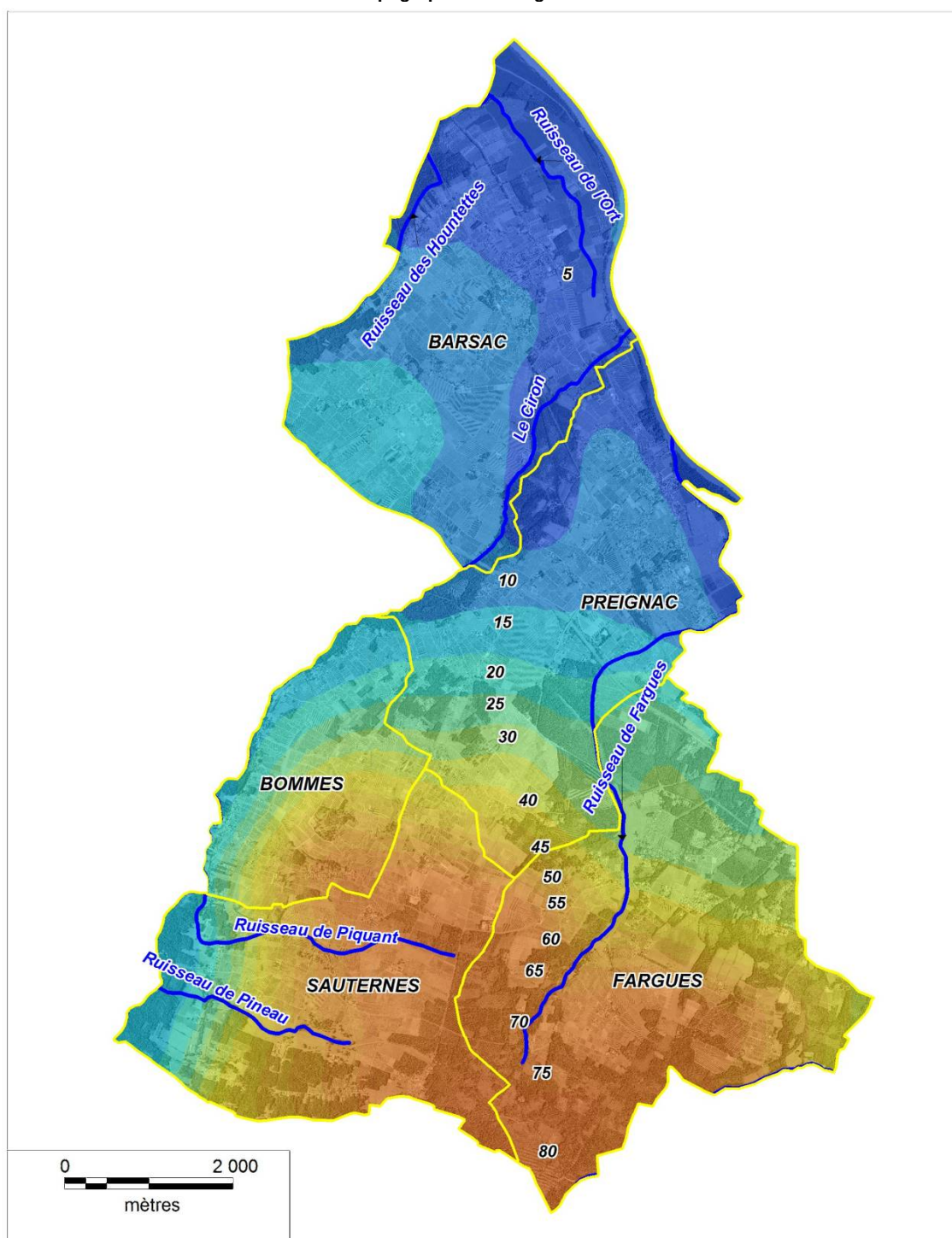
Carte 2 : Topographie de la région de Sauternes
