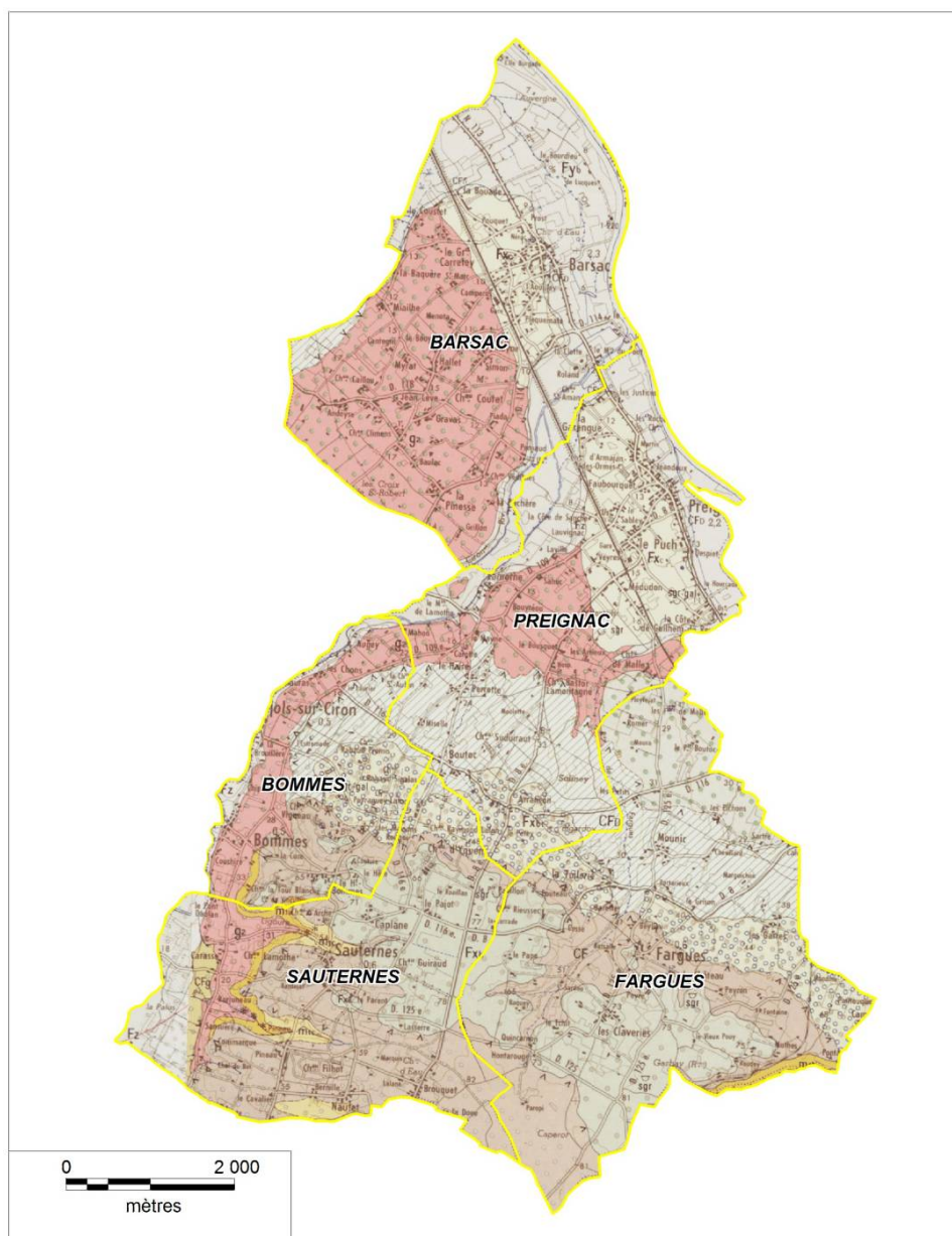
Carte 4 : Géologie simplifiée d'après BRGM au 1/50 000
