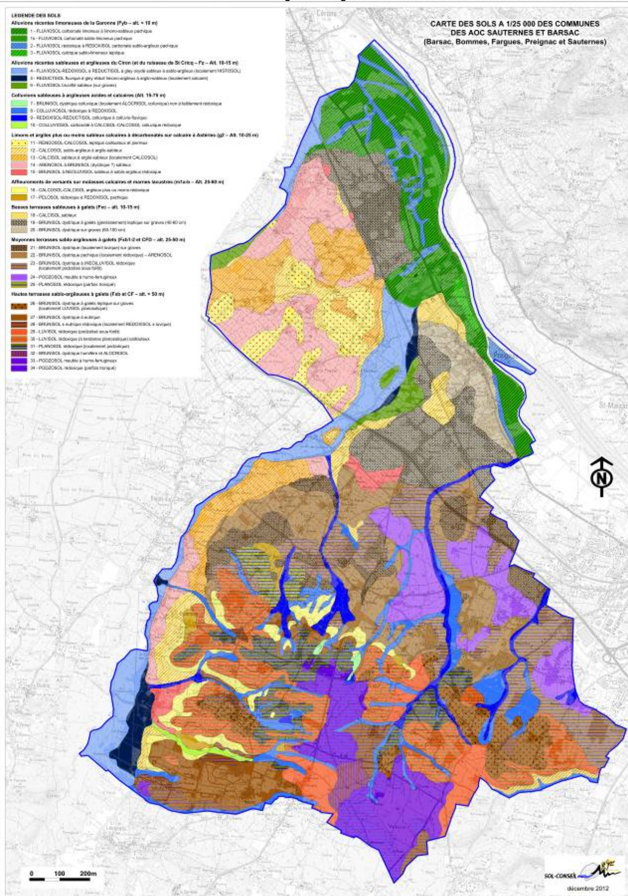
Carte 1 : Pédologie de la région de Sauternes
